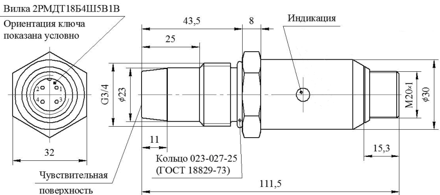
Рис.2 - Габаритный чертеж
