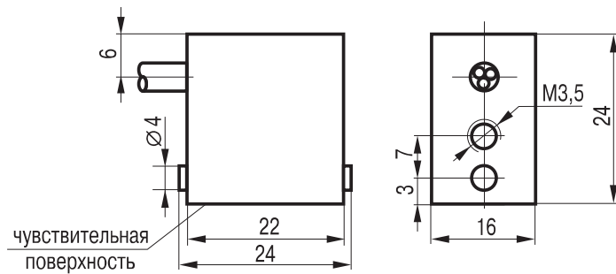
Габаритный чертеж
