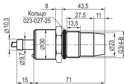
Схема монтажа
