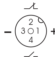
Цоколевка соединителя (вид со стороны монтажа)
