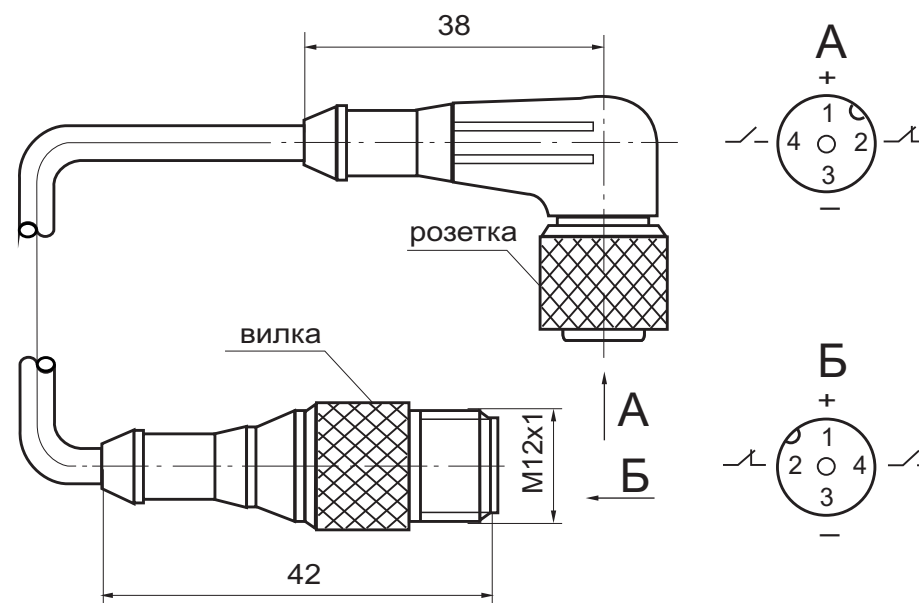
Габаритный чертёж
