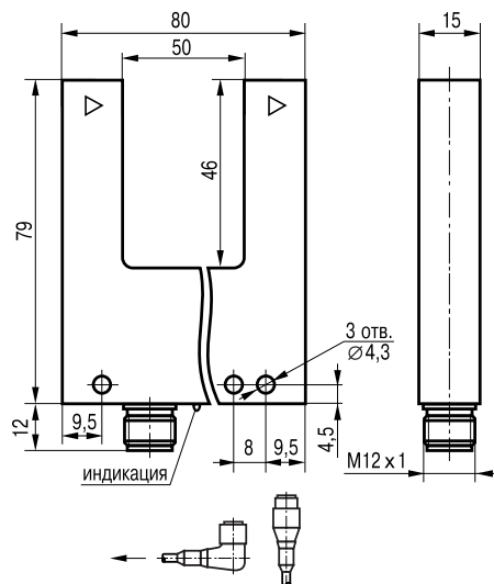
Габаритный чертёж
