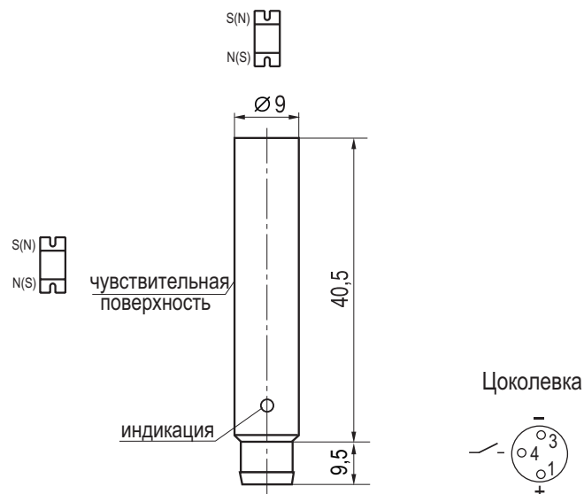
Габаритный чертеж
