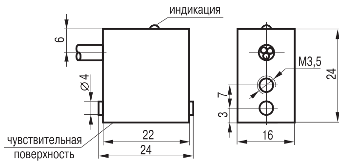
Габаритный чертёж
