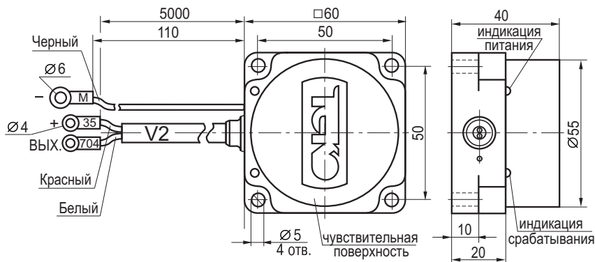
Габаритный чертеж
