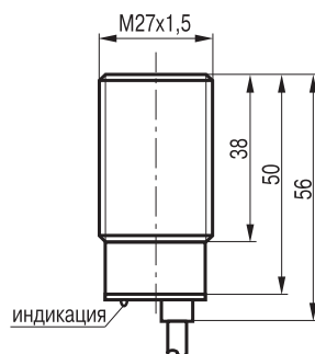
Габаритный чертеж
