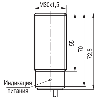
Габаритный чертеж
