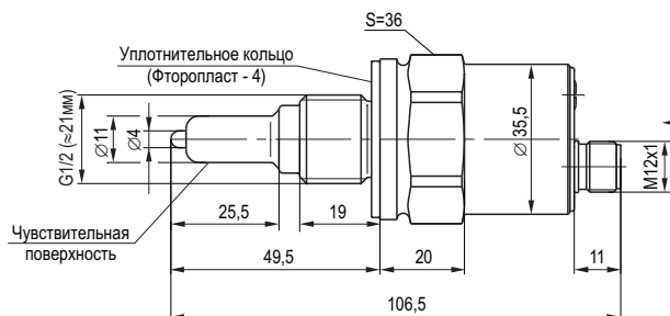
Габаритный чертеж.
