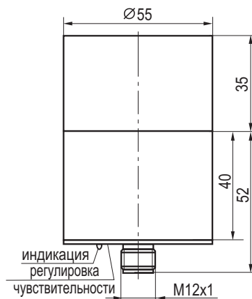
Габаритный чертеж
