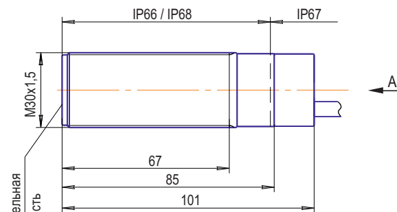
Габаритный чертеж
