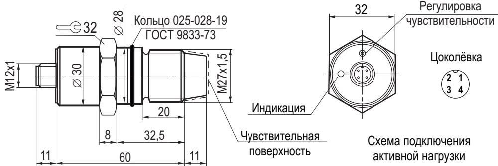
Схема монтажа
