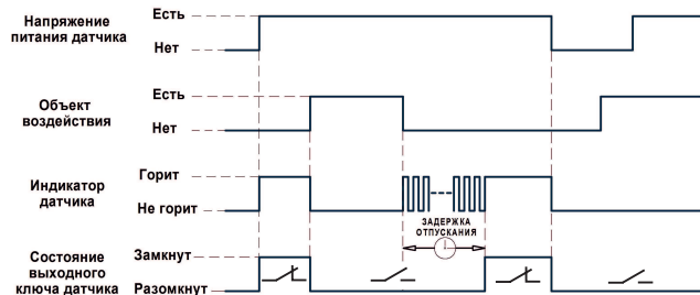
Диаграмма работы датчика
