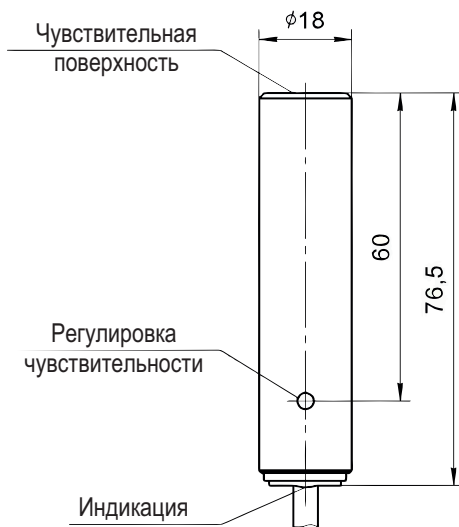
Габаритный чертеж
