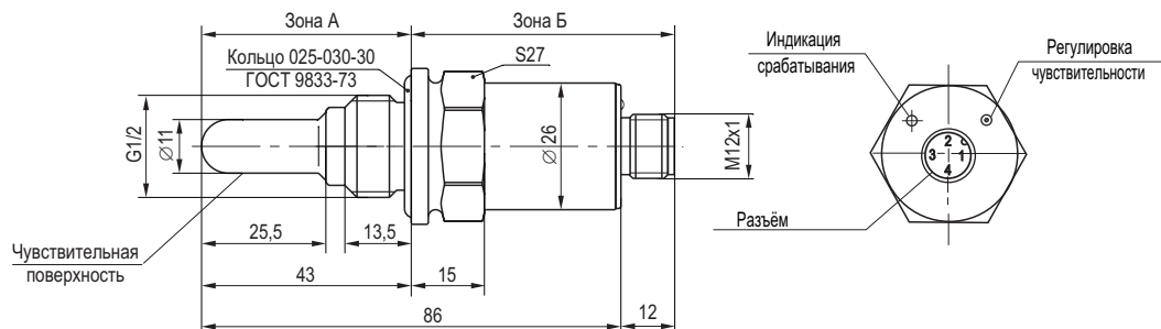
Габаритный чертёж
