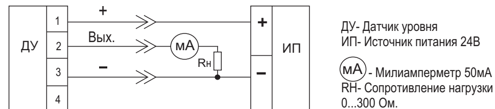
Рис.2. Схема подключения датчика уровня CSA EC49A8-32P-500-PR18
