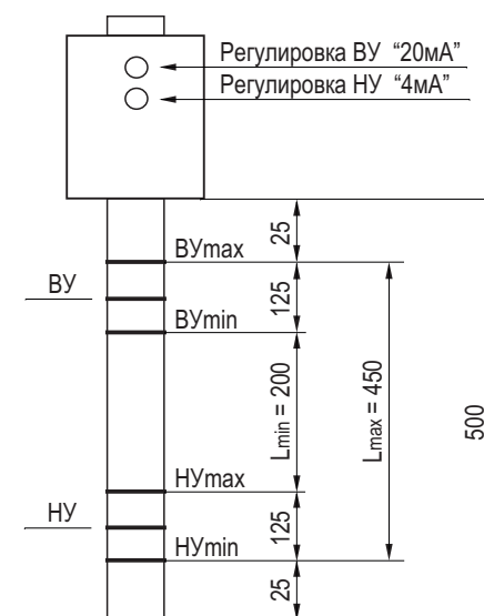
Рис.1. Датчик уровня CSA EC49A8-32P-500-PR18
