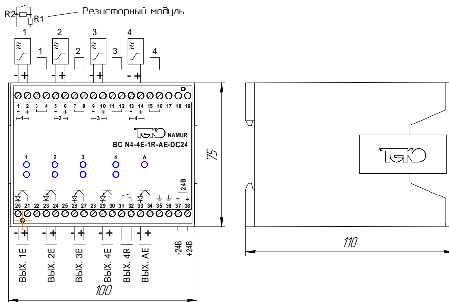
ГАБАРИТНЫЙ ЧЕРТЕЖ СХЕМА ПОДКЛЮЧЕНИЯ БЛОКА СОПРЯЖЕНИЯ
